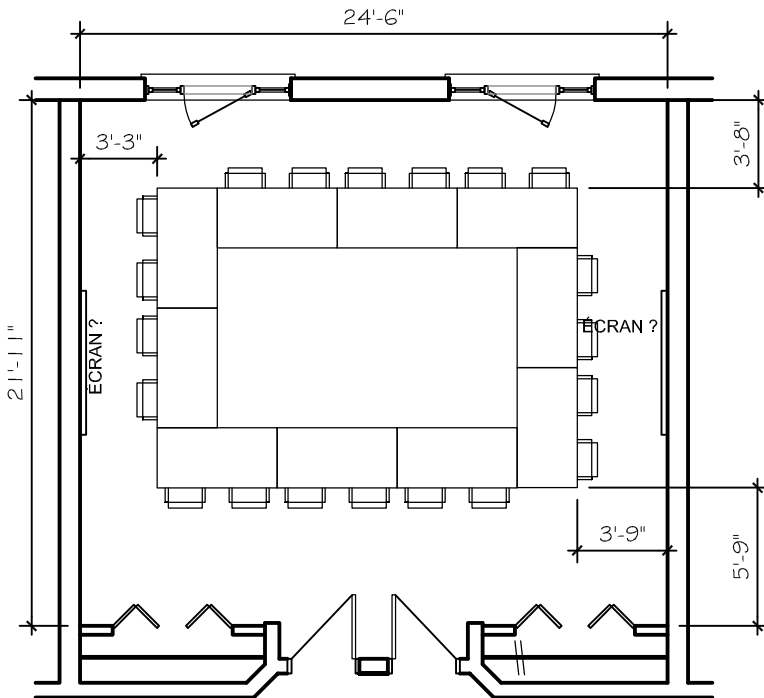
Salle Multi-Média 103-105 échelle: 1/4" = 1'-0" Aménagement CARRÉ (avec tables de 30"x60") 20 personnes
